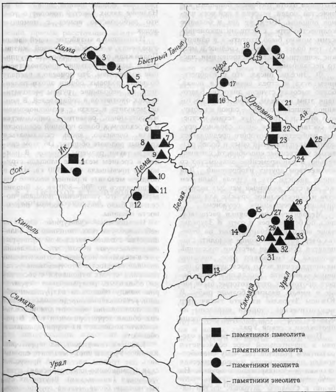
Карта I. Расположение основных памятников эпохи камня на Южном Урале
